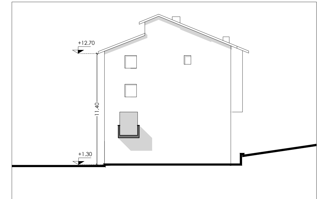
PROFILO NORD OVEST 1:200
