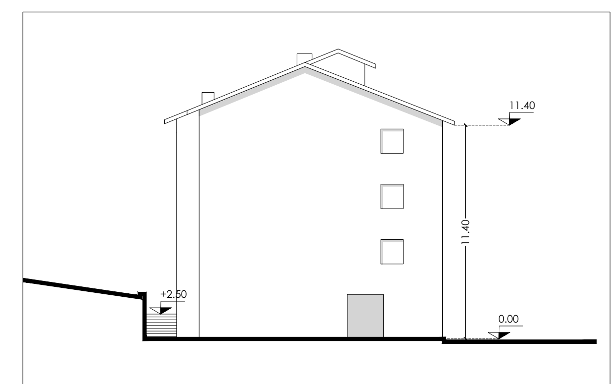
PROFILO SUD EST_Scala 1:200
