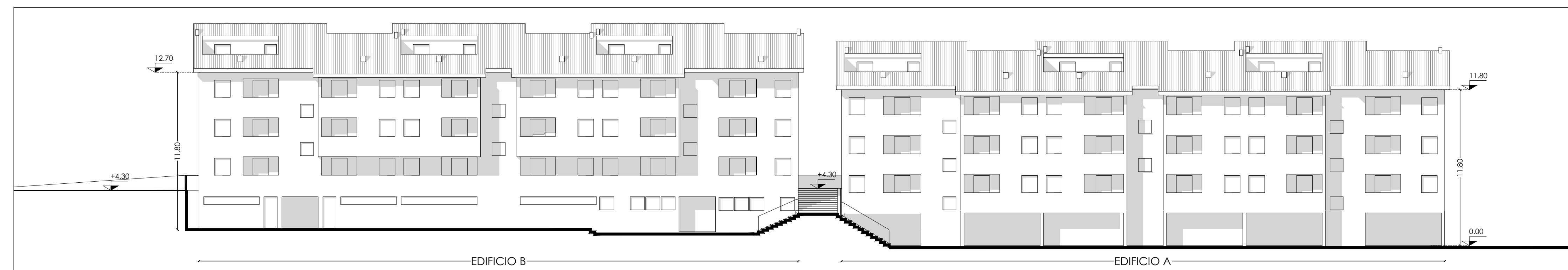
PROFILO SUD OVEST_Scala 1:200
